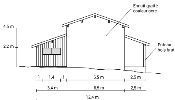
FAÇADE OUEST
